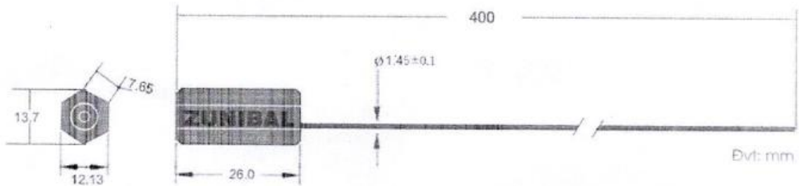
Hình 1. Thông số kỹ thuật của dây niêm phong
