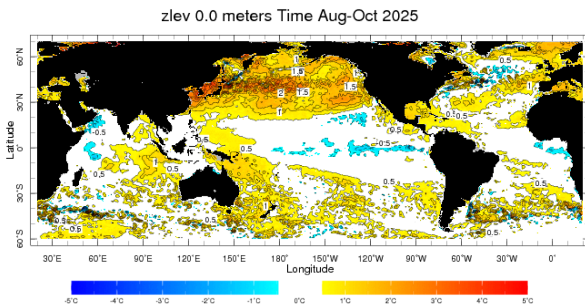
Hình 1.1. Phân bố chuẩn sai nhiệt độ mặt nước biển trung bình mùa 3 tháng 8-10 năm 2025 (°C)
