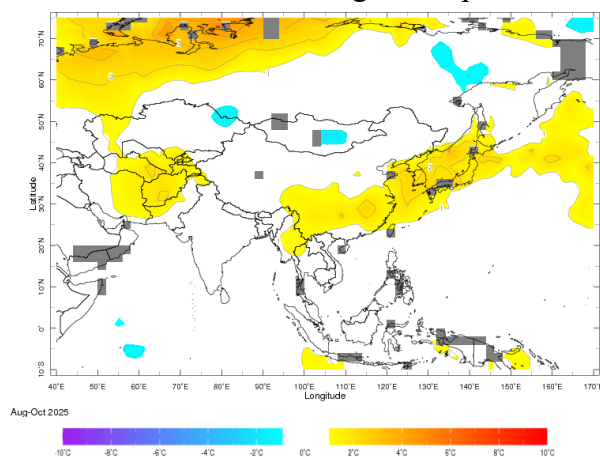
Hình 1.4. Phân bố chuẩn sai NĐTB mùa 3 tháng 8-10 năm 2025 (°C) trên khu vực châu Á (Nguồn: http://iridl.ldeo.columbia.edu/ )
