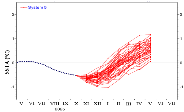
Hình 2.2. Dự báo SSTA tại khu vực NINO3.4 mùa 3 tháng 12-02 năm 2025/2026
