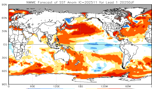
Hình 2.1. Dự báo SSTA mùa 3 tháng 12-02 năm 2025/2026
