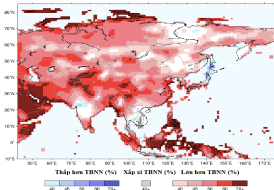
Hình 2.3. Dự báo xác suất nhiệt độ mùa 3 tháng 12-02 năm 2025/2026 cho khu vực châu Á
