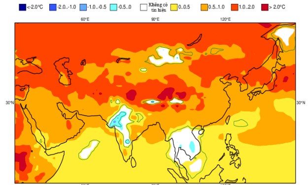
Hình 2.4. Dự báo chuẩn sai nhiệt độ mùa 3 tháng 12-02 năm 2025/2026
