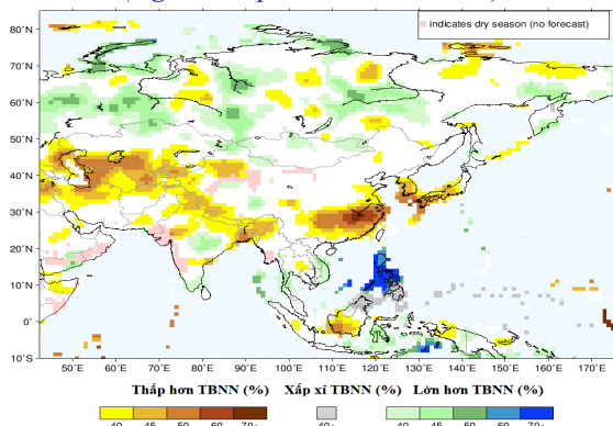
Hình 2.5. Dự báo xác suất lượng mưa mùa 3 tháng 12-02 năm 2025/2026 cho khu vực châu Á
