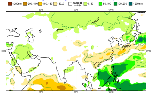
Hình 2.6. Dự báo chuẩn sai lượng mưa mùa 3 tháng 12-02 năm 2025/2026
