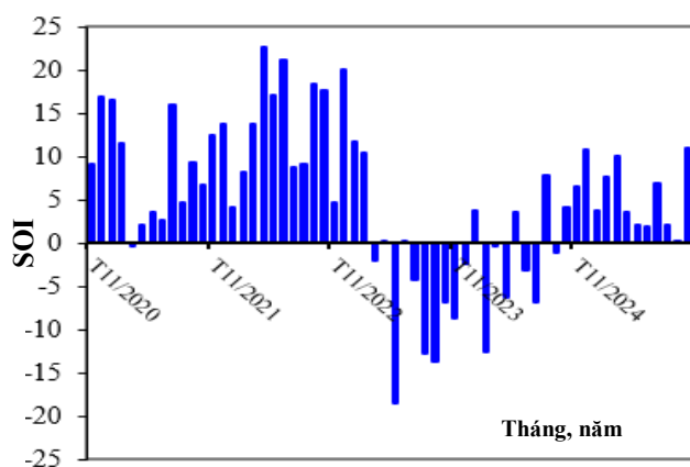
Hình 1.2. Diễn biến chỉ số SOI (11/2020 - 10/2025)
